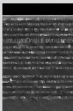
TiO 2 /SiO 2 多層膜の断面SEM画像
