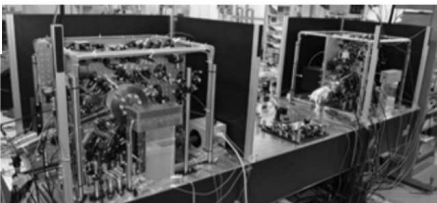
光格子時計 © 2015 齋取秀俊
